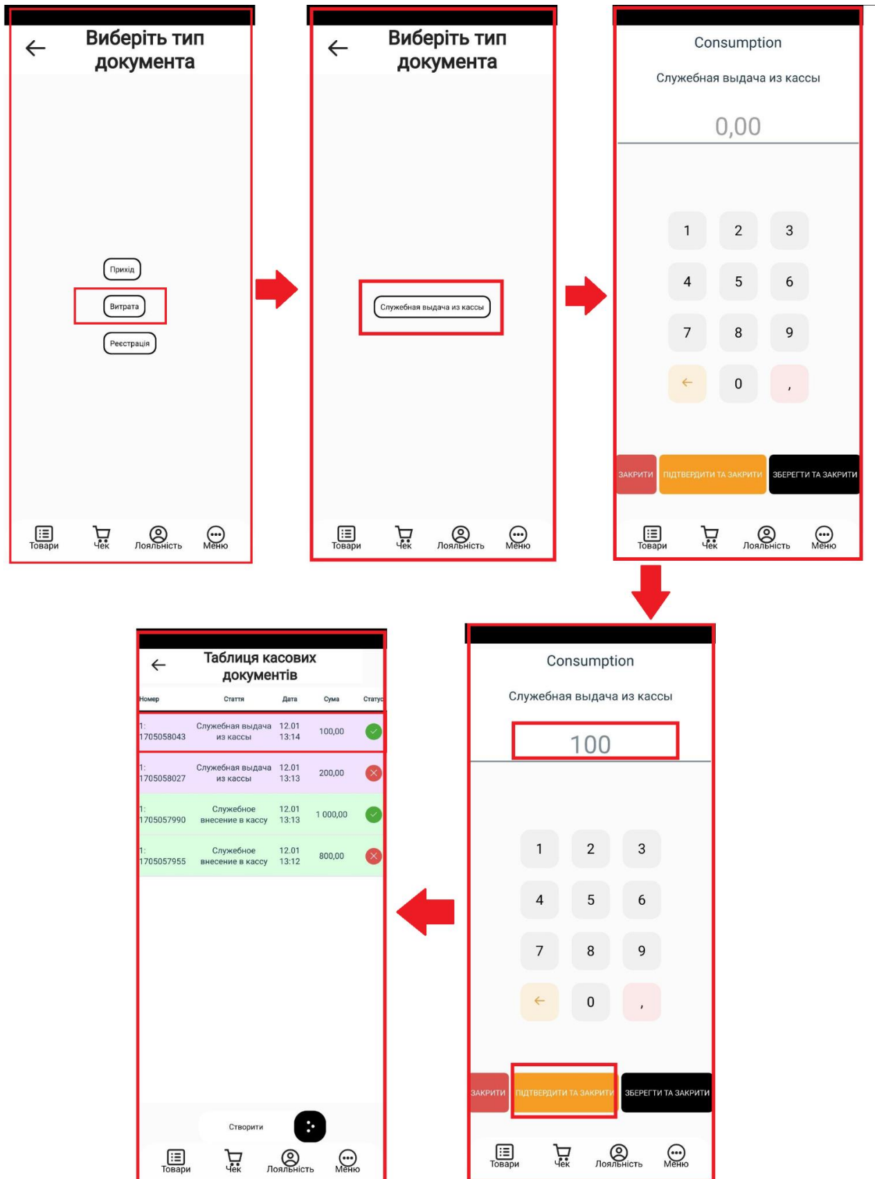
Рисунок 66 - Створення та відображення вже створеного касового документа "Витрата" у статусі "Проведений"
