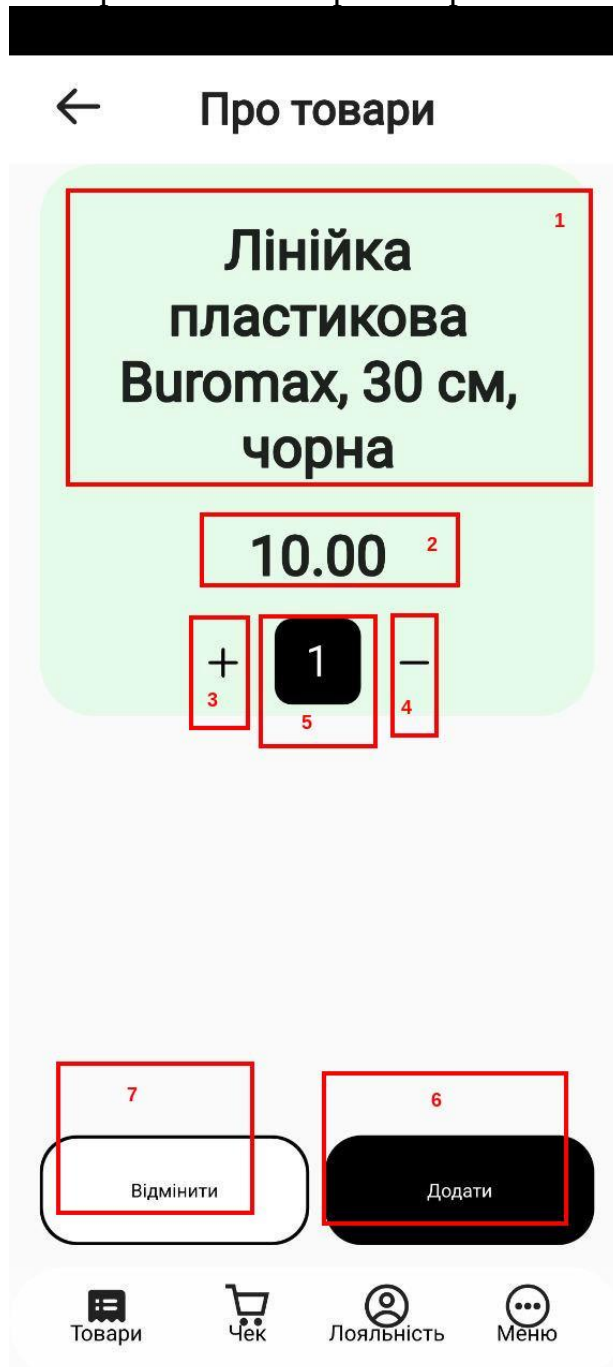
Рисунок 17 - Результат натискання на товар - поява вікна “Про товари” з обраним товаром із каталогу товарів.
