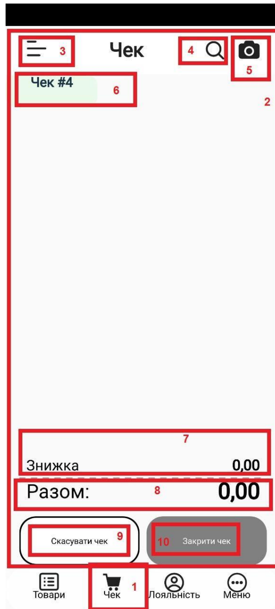
Рисунок 95 - Інтерфейс вікна “Чек”
