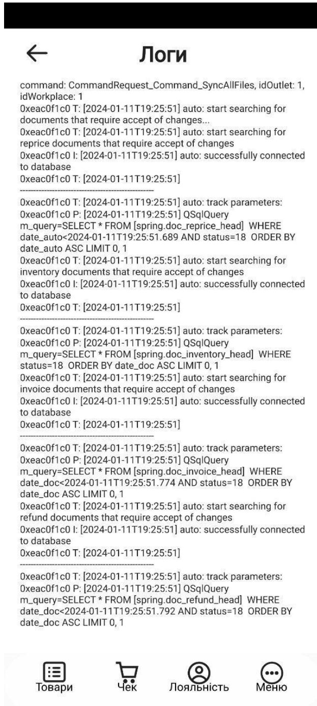
Рисунок 88- Відображення логів при натисканні на кнопку “Показати журнал логування”
